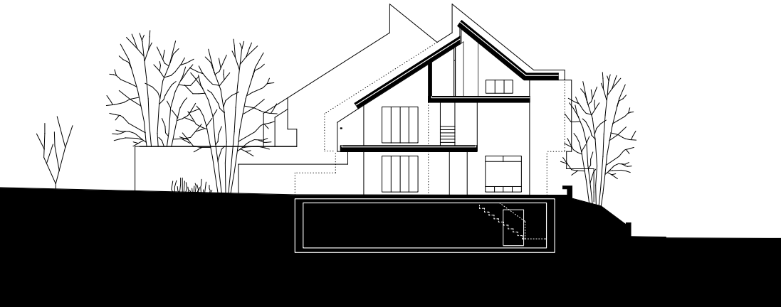
Schnitt A 1:300
