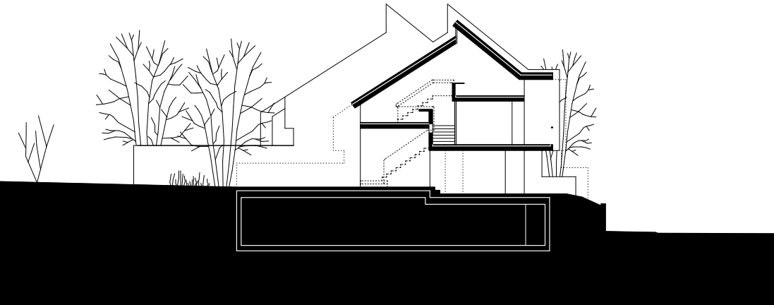
Schnitt B 1:300
