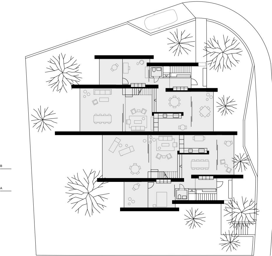
Erdgeschoss 1:300
